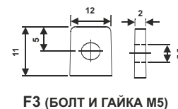
F3 (БОЛТ И ГАЙКА M5)
